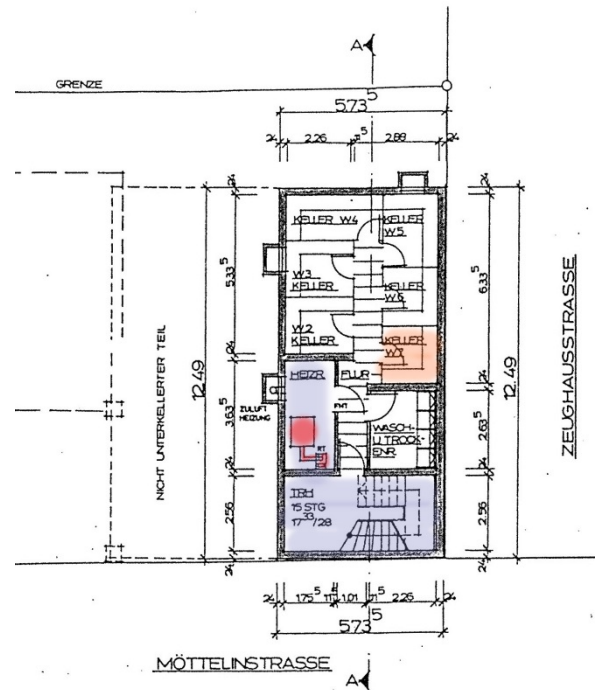
UNTERGESCHOSS
