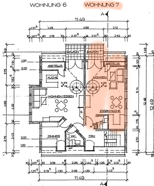
DACHGESCHOSS
