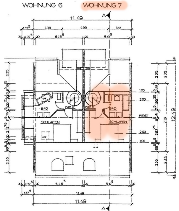
DACHSPITZ
